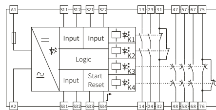
CZSR8001-2A1B3AT1BT
